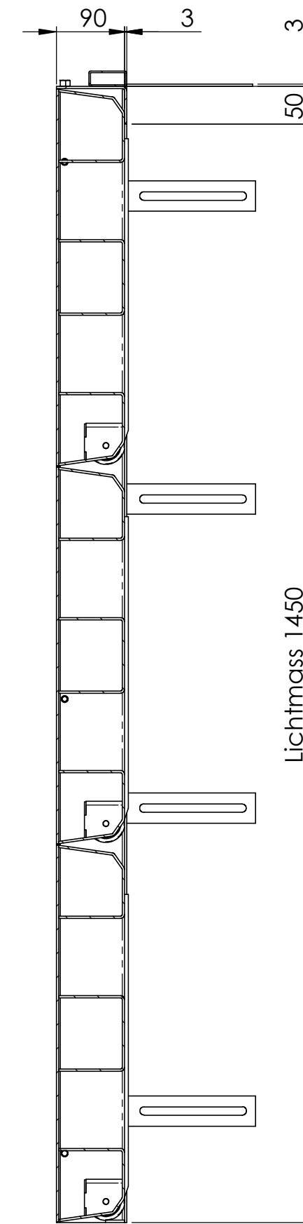
SCHNITT B-B MABSTAB 1:7
